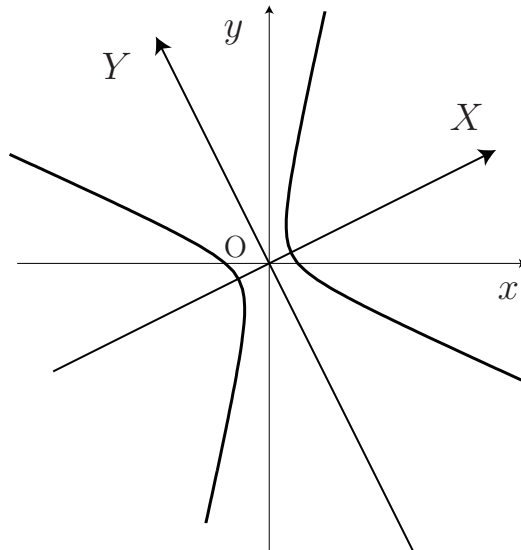
図 1: 2x^2 + 4xy - y^2 = 1 の概形
