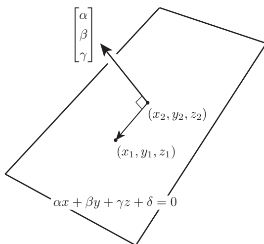
図 2: 平面と法線ベクトル
